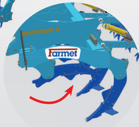
mechaniczne odchylenie jednego rzędu
