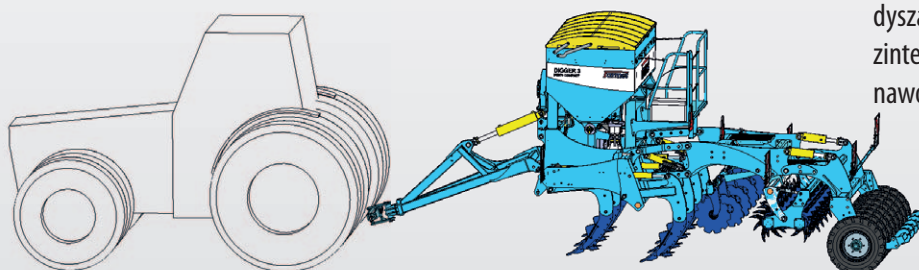
Digger P FW | uzupełniający nośnik z osią, zasobnik nawozu, nawożenie do 2 poziomów
