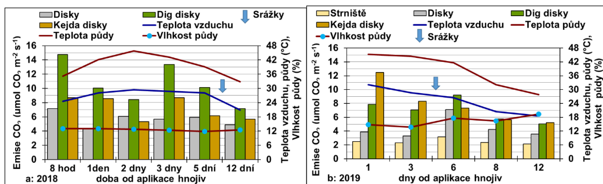
Obr. 91: Emise \text{CO}_2 po zapravení povrchově aplikované kejdy a digestátu.
