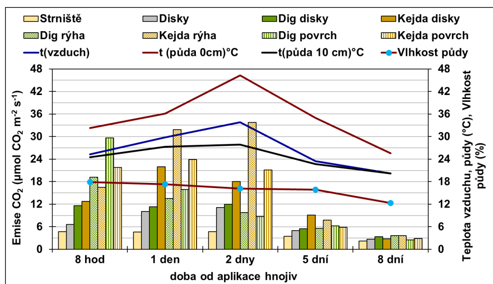
Obr. 92: Emise CO 2 po různých způsobech aplikace a zapravení digestátu a kejdy (2020).
