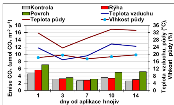
Obr. 90: Emise CO 2 po přihnojení porostu kukuřice digestátem v roce 2020.
