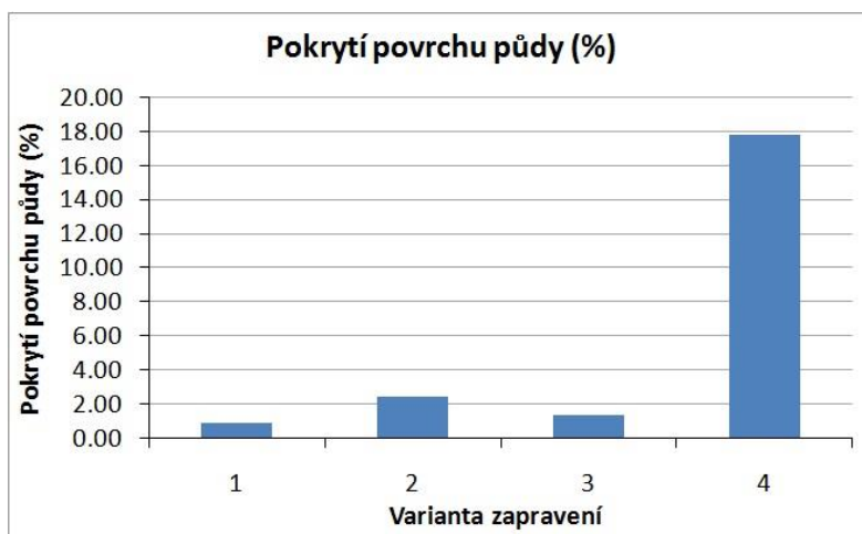
Obr. 52: Pokrytí povrchu půdy modrou barvou po aplikaci. Číslo 1 odpovídá technickému řešení a), 2 – b); 3 – d) a 4 – c) – viz. obrázek 48.
