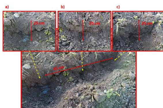
Obr. 44: Rozmístění kejdy v půdním profilu v závislosti na způsobu nastavení hloubky křídel (foto Brant).
