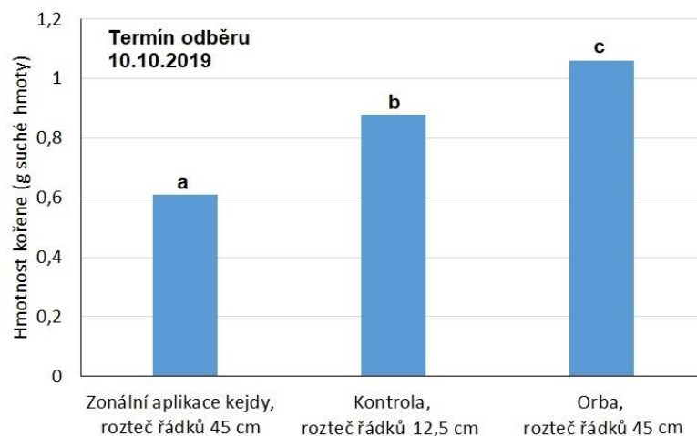
Obr. 76: Průměrné hmotnosti kořenů pro jednotlivé varianty. Statisticky významné rozdíly na hladině významnosti 0,05 (ANOVA, Tukey) jsou vyznačeny rozdílnými indexy.
