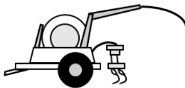
Obr. 7: Technické možnosti eliminace utužení půdy při aplikaci tekutých hnojiv (Brant a kol., 2017).
