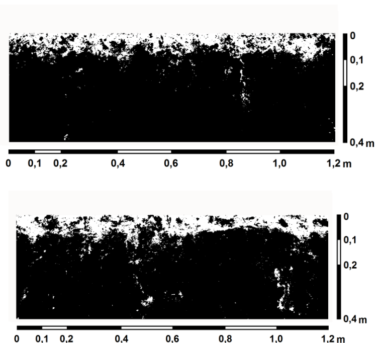
Obr. 65: Profily na obrázcích přináší pohled na variantu s plošnou aplikací kejdy. Horní obrázek dokumentuje infiltraci po zalití modrou barvou 25.11.2019. Z obrázku je patrná nižší intenzita infiltrace do půdy. Na profilu jsou patrné stopy po hlubším kypření, které bylo provedeno v předchozích letech. Nicméně pro infiltraci byla limitující utužená vrstvě v hloubce zpracování půdy. Dole je stav infiltrace 24 hodin po zalití modrou barvou.
