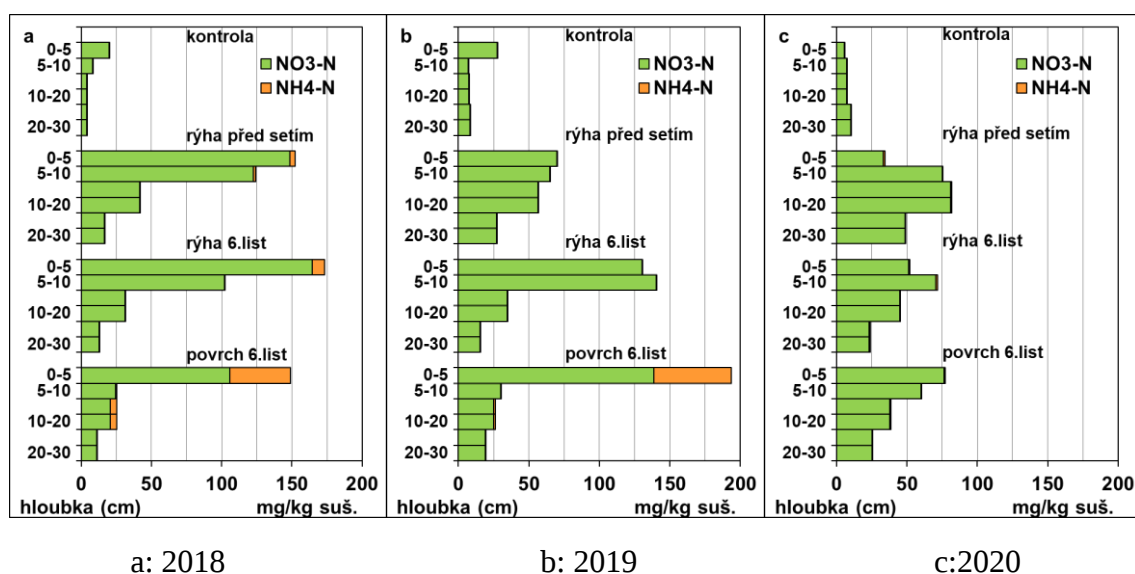
Obr. 98: Rozdělení N_{min.} v půdě v místě aplikace (odběr byl proveden ve fázi 10. listu).
