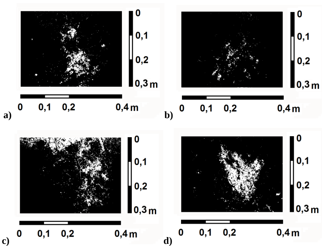
Obr. 49: Profil půdy, který byl odkryt kolmo na směr jízdy, dokládá vliv umístění koncovek aplikátorů na rozptyl obarvené vody v profilu půdy, označení a) – d) vychází z údajů uvedených na obrázku 21. Bílá barva dokumentuje přítomnost modré barvy.
