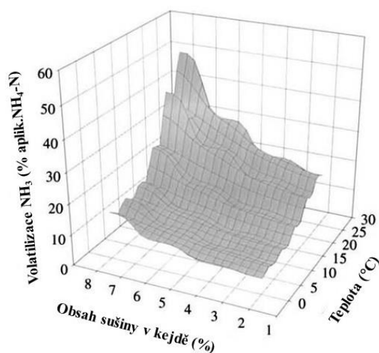
Obr. 2: Volatilizace amoniaku ve vztahu k obsahu sušiny v kejdě a teplotě (Sommer a Hutchings, 2001).
