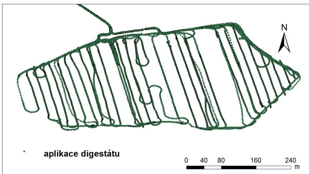
Obr. 11: Záznam přejezdů při aplikaci digestátu. Některé části pozemku jsou vystaveny vysoké zátěži od kol.
