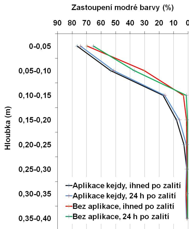
Obr. 66: Rozdíly v intenzitě infiltrace mezi jednotlivými variantami. Statisticky významné rozdíly pro jednotlivé varianty byly hledány pomocí analýzy rozptylu.
