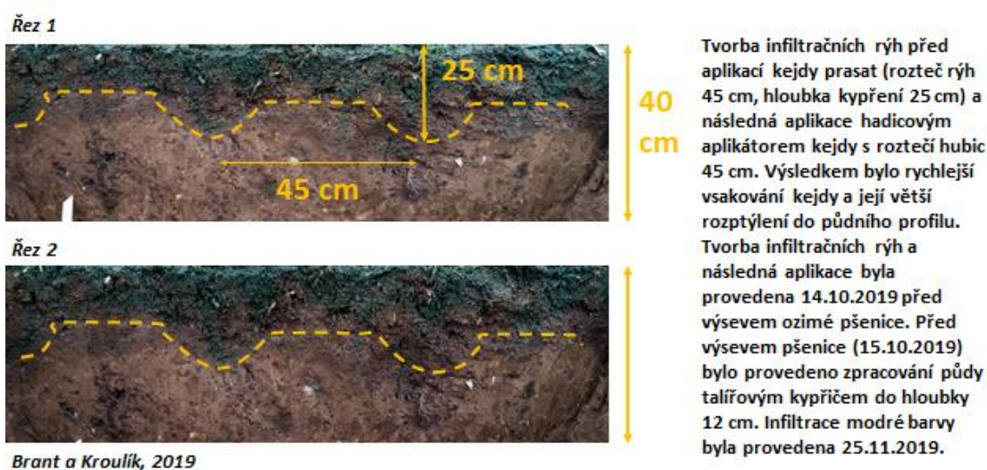
Obr. 63: Hodnocení infiltrace modré barvy na plochách s tvorbou infiltračních rýh.
