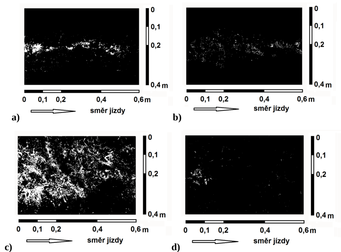
Obr. 51: Zejména u varianty 4 (vpravo dole), je patrné, že větší vzdálenost od pracovních nástrojů a zakončení hadice usměrňovací deskou vedlo k výraznému omezení zaklopení hnojiva. Bílá barva dokumentuje přítomnost modré barvy.
