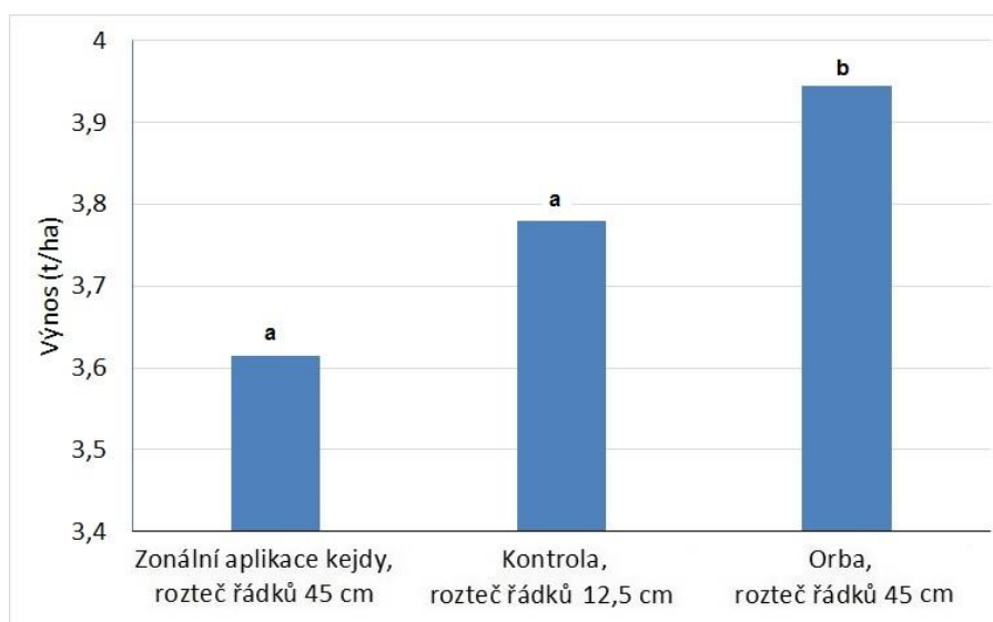
Obr. 82: Výnos semene řepky pro jednotlivé varianty. Statisticky významné rozdíly na hladině významnosti 0,05 (ANOVA, Tukey) jsou vyznačeny rozdílnými indexy.
