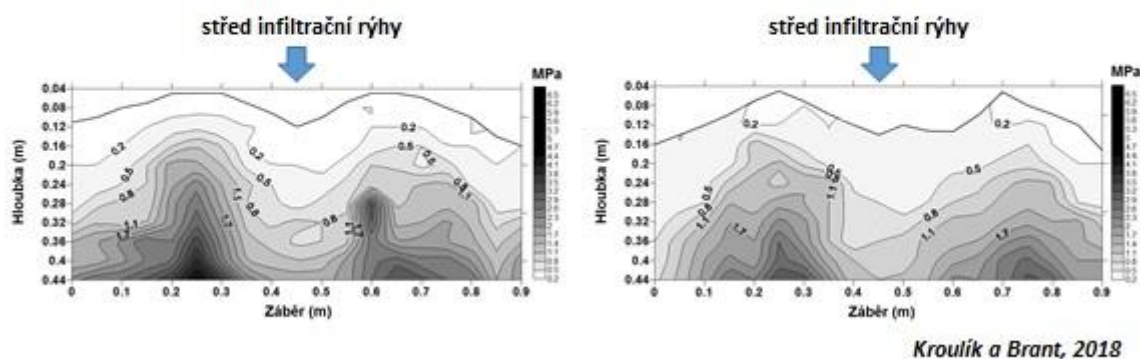
Obr. 30: Hodnoty penetračního odporu půdy v závislosti na šířce kypřicího dlátka.
