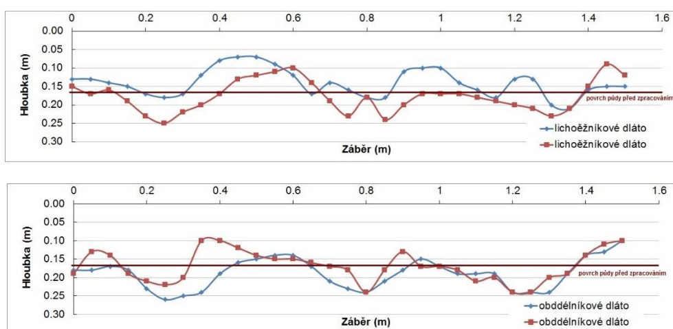
Obr. 33: Hodnoty kolmého průmětu povrchu půdy vůči směru pracovní jízdy v závislosti na použitém pracovním nástroji - dláto lichoběžníkového (nahore) a obdélníkového tvaru (dole).
