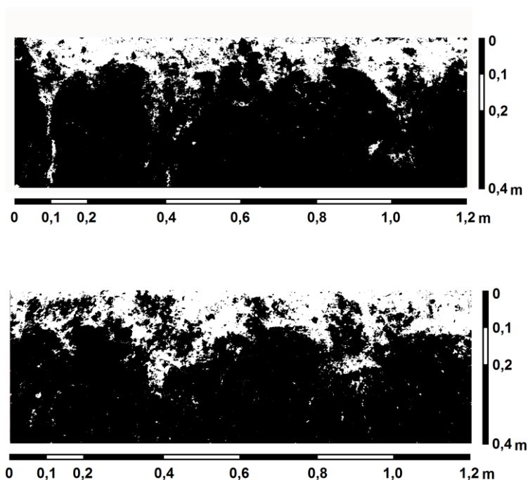
Obr. 64: Profil na pozemku s vytvořenými infiltračními rýhami, odkrytý ihned po zalití 25.11.2019 (nahore) s dobře patrnými infiltračními rýhami. Dole je znázorněn profil na pozemku s vytvořenými infiltračními rýhami, odkrytý 24 hodin po zalití. Na prezentovaných řezech je rovněž parná přítomnost infiltračních rýh.
