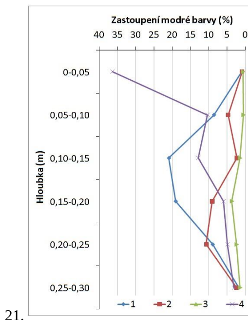
Obr. 50: Vliv technického řešení aplikace kapaliny na intenzitu infiltrace a zapravení modré barvy do půdy. Číslo 1 odpovídá technickému řešení a), 2 – b); 3 – d) a 4 – c) – viz. obrázek 48.
