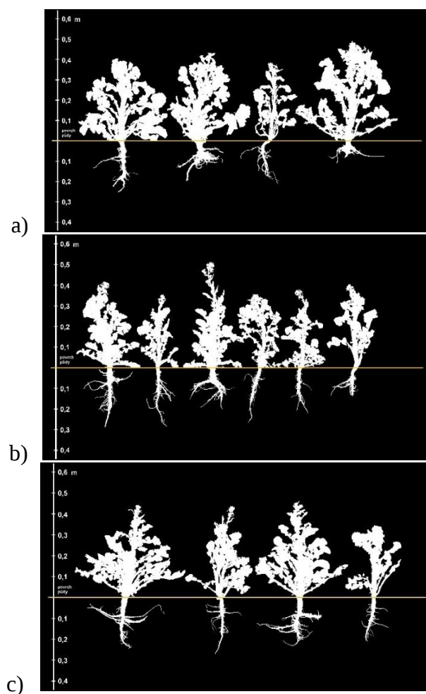
Obr. 81: Obrázky rostlin odebraných z jednotlivých variant. Varianty: a) zonální aplikace kejdy a rozteč řádků 0,45 m; b) kontrolní varianta s roztečí 0,125 m; c) varianta s orbou a s roztečí řádků 0,45 m.
