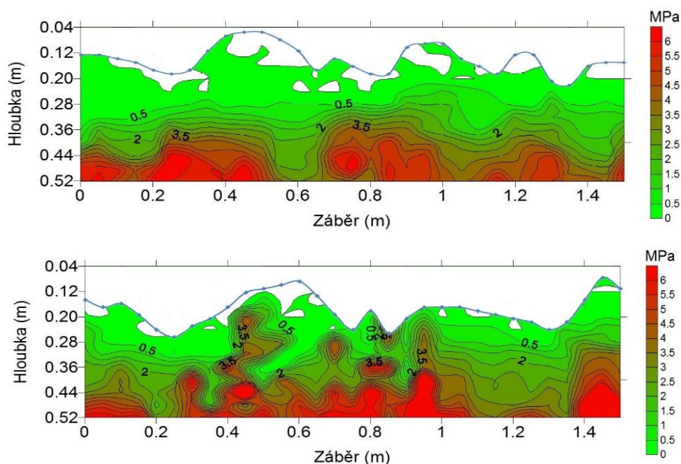
Obr. 31: Vliv kypřicího dlátka lichoběžníkového tvaru na hodnoty penetračního odporu půdy.
