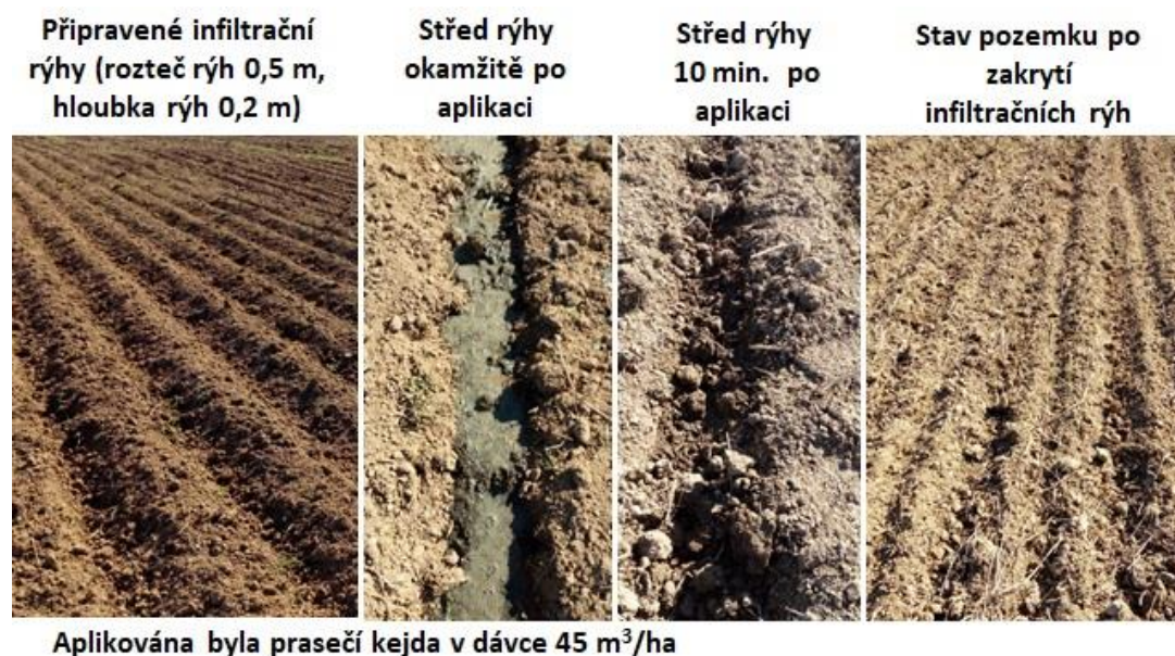
Obr. 36: Stav pozemku po provedení tvorby infiltračních rýh, po aplikaci kejdy prasat a po zahrnutí infiltračních rýh.
