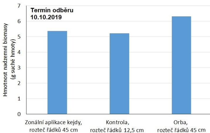
Obr. 77: Průměrné hmotnosti nadzemních částí rostlin pro jednotlivé varianty. Statisticky významné rozdíly nebyly nalezeny.
