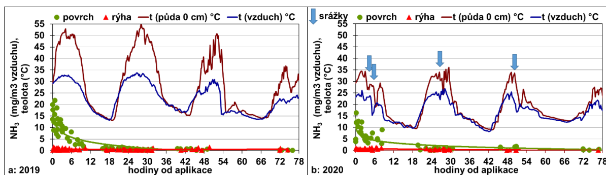
Obr. 87: Koncentrace amoniaku ve vzduchu po přihnojení kukuřice digestátem.
