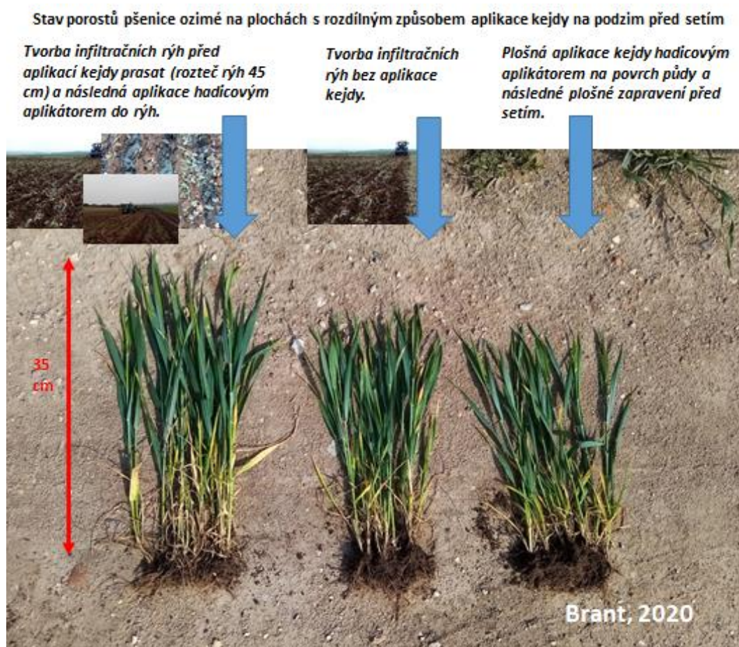
Obr. 70: Stav porostů na hodnocených plochách 15.5.2020.
