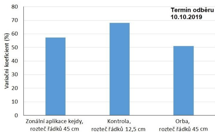
Obr. 75: Pravidelnost rozmístění rostlin v řádku, vyjádřená variačním koeficientem.
