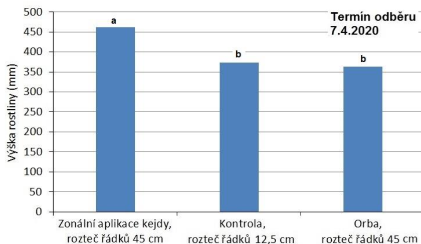
Obr. 80: Průměrné hodnoty výšek nadzemních částí rostlin. Statisticky významné rozdíly na hladině významnosti 0,05 (ANOVA, Tukey) jsou vyznačeny rozdílnými indexy.
