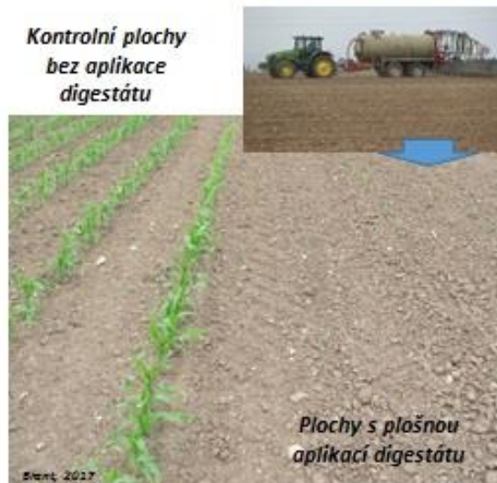
Obr. 9: Stav porostů kukuřice na plochách s plošnou aplikací digestátu a bez aplikace. Utužení půdy vedlo k tvorbě velkých půdních agregátů, a tím ke snížení množství vody v horní vrstvě půdy, což výrazně zpomalilo i růst rostlin.
