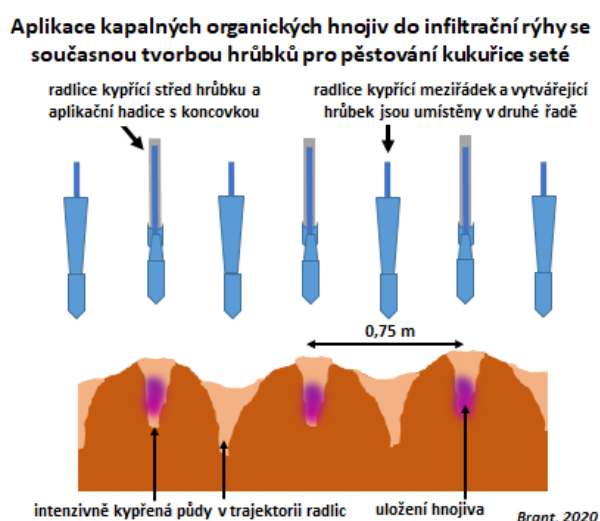
Obr. 53: Systémy aplikace kapalných organických hnojiv do vertikálních infiltračních rýh lze uplatnit i v systémech pěstování širokořádkových plodin v hrůbcích.
