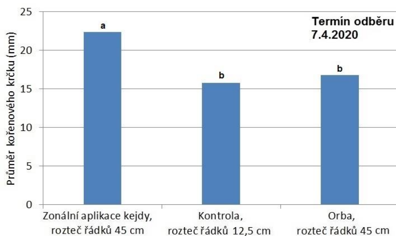
Obr. 79: Průměrné hodnoty průměrů kořenového krčku. Statisticky významné rozdíly na hladině významnosti 0,05 (ANOVA, Tukey) jsou vyznačeny rozdílnými indexy.
