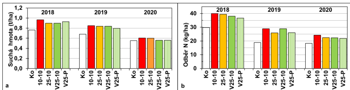
Obr. 99: Nadzemní hmota rostlin a příjem dusíku ve fázi 10. listu po různém způsobu aplikace digestátu.
