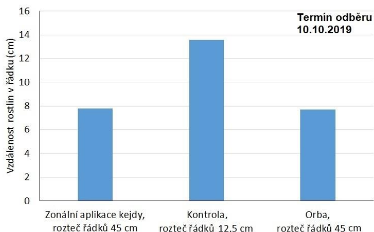
Obr. 74: Rozteče rostlin v řádcích pro jednotlivé varianty.
