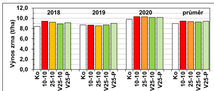
Obr. 100: Výnos zrna kukuřice po různém způsobu aplikace digestátu.
