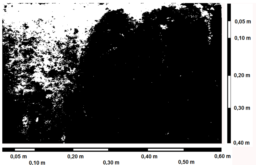
Obr. 10: Vliv přejezdu kola traktoru na infiltraci vody do půdy v porostech kukuřice před sklizní (pravá část obrázku). Bílá barva znázorňuje infiltraci vody a černá půdu.
