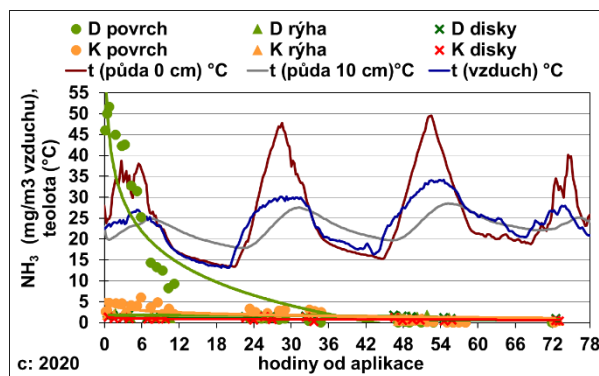
Obr. 89: Koncentrace amoniaku ve vzduchu po různé aplikaci digestátu a kejdy na slámu.
