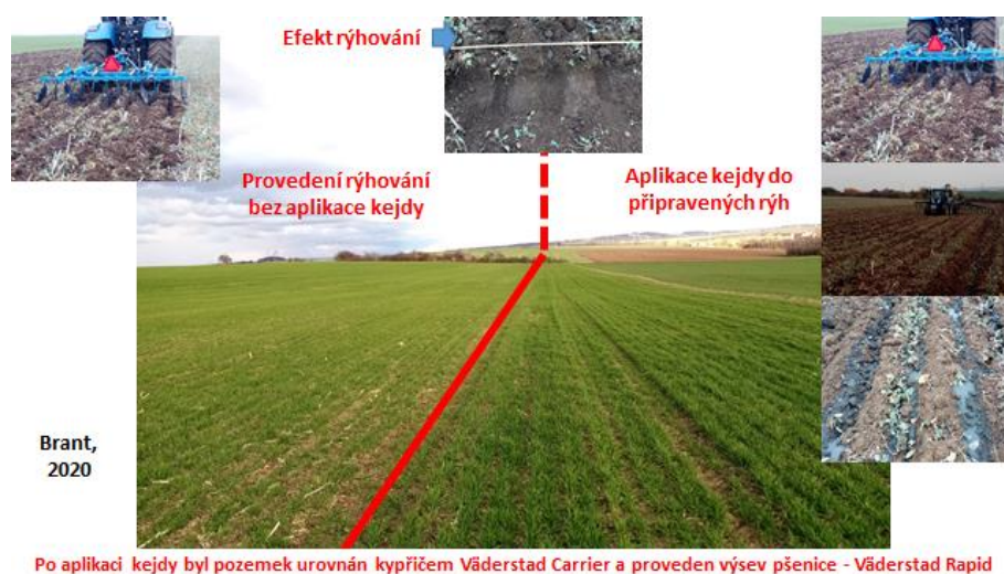
Obr. 69: Stav porostů ozimé pšenice 13.3.2020 na plochách s tvorbou infiltračních rýh s aplikací a bez aplikace kejdy.
