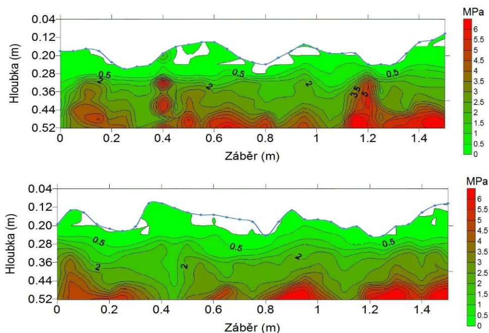
Obr. 32: Vliv kypřicího dláta obdélníkového tvaru na hodnoty penetračního odporu půdy.
