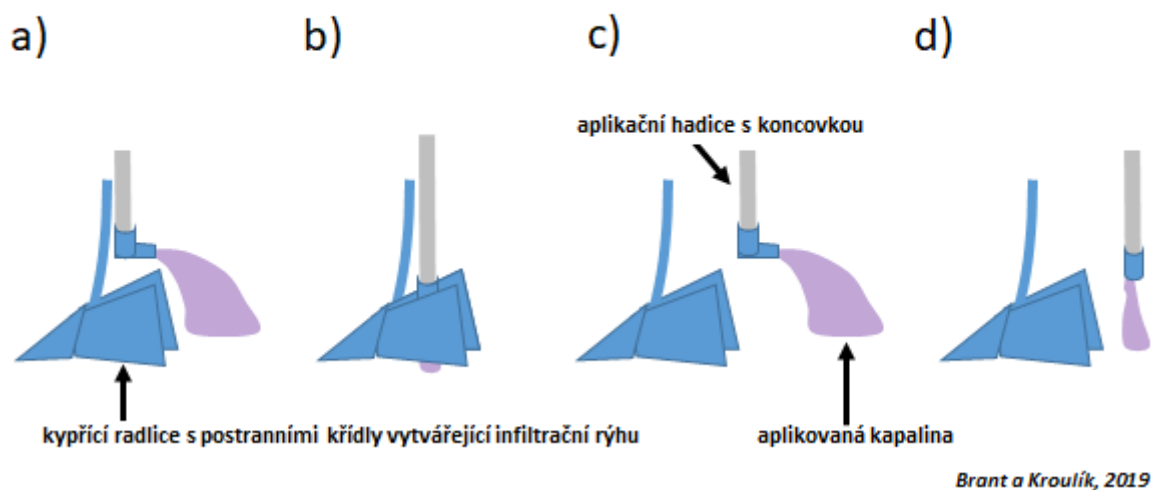
Obr. 48: Rozdílné systémy aplikace kapalných organických hnojiv za kypřicí radlice.
