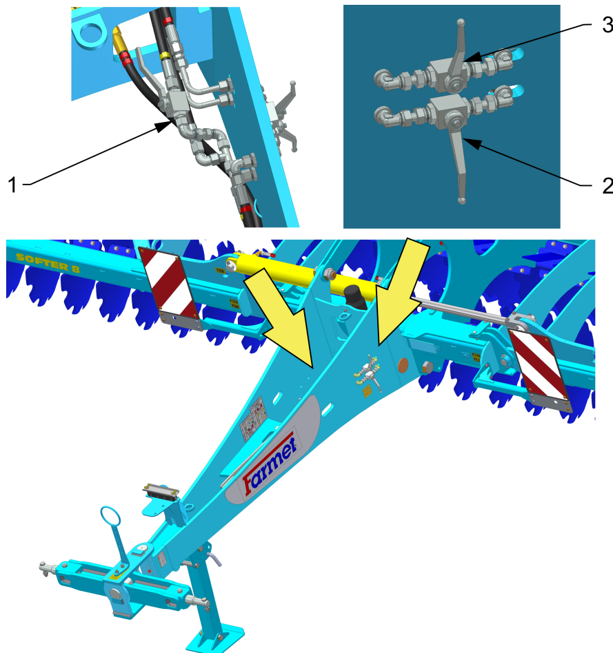
Abb. 2 - Absperrventile (Kugelventile)
