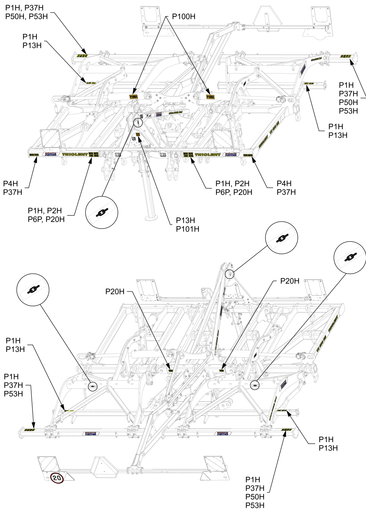
Obr. 1 - Umístění bezpečnostních štítků na stroji TRIOLENT TX 400 NS
