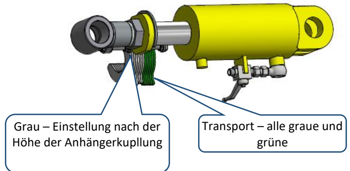
Abb. 15 Unterlagen der Kolbenstange der Deichsel
