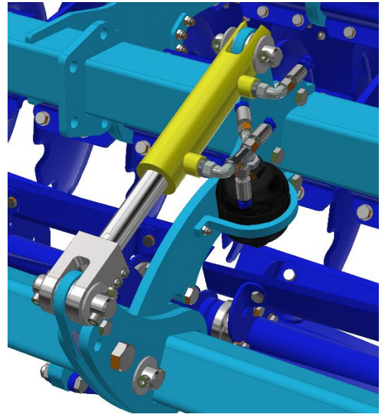
Abb. 17 Kolbenstange des vorderen Werkzeugs
