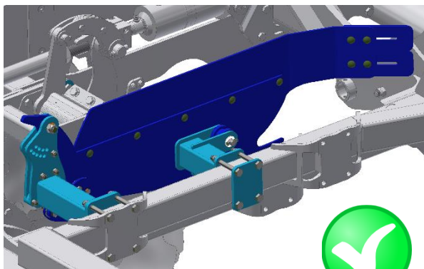
Abb. 9 Richtiges Umklappen der Abweiser
