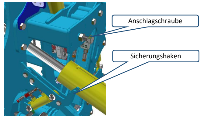
Abb. 28 Anschläge der Seitenrahmen
