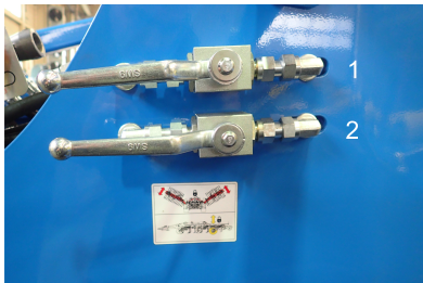
Abb. 2 - Absperrventile (Kugelventile)
