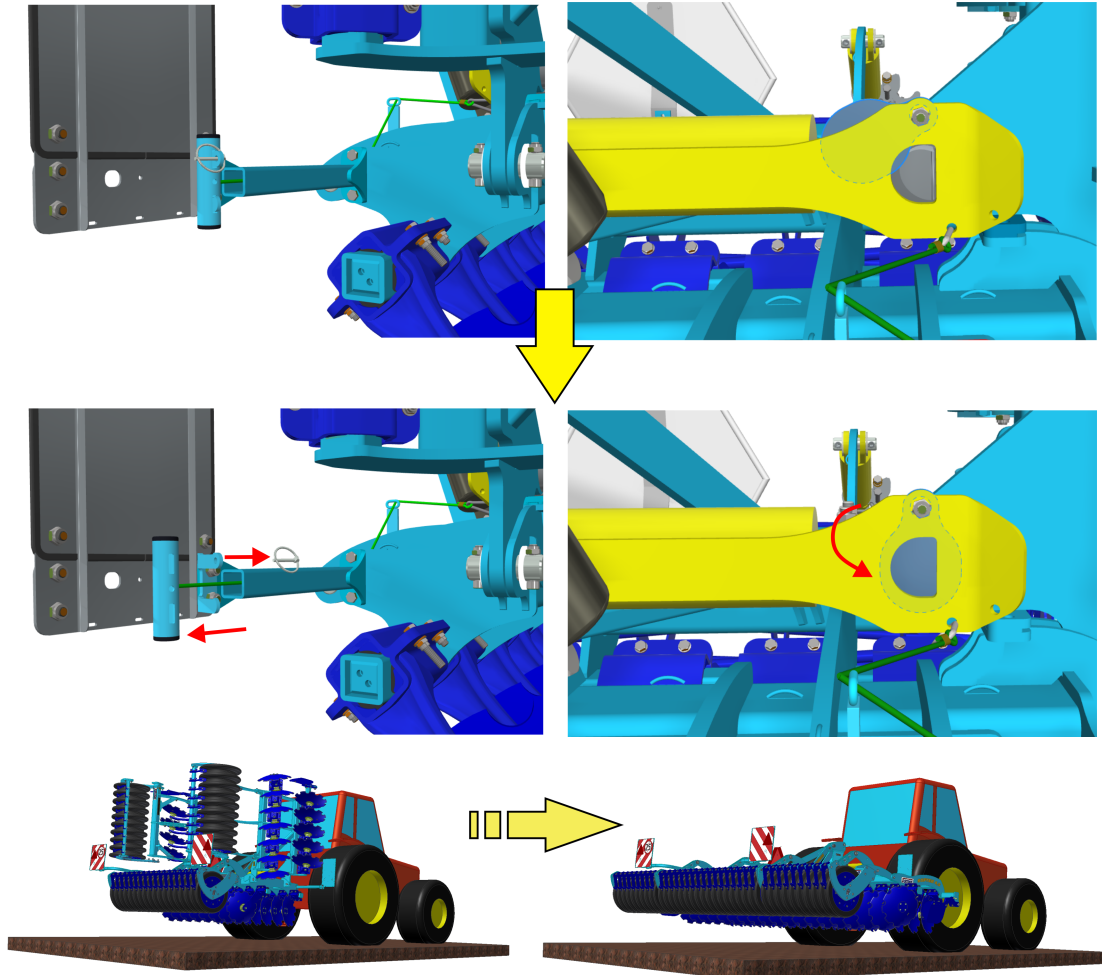
Rys. 2 - Odblokowanie cięgna
