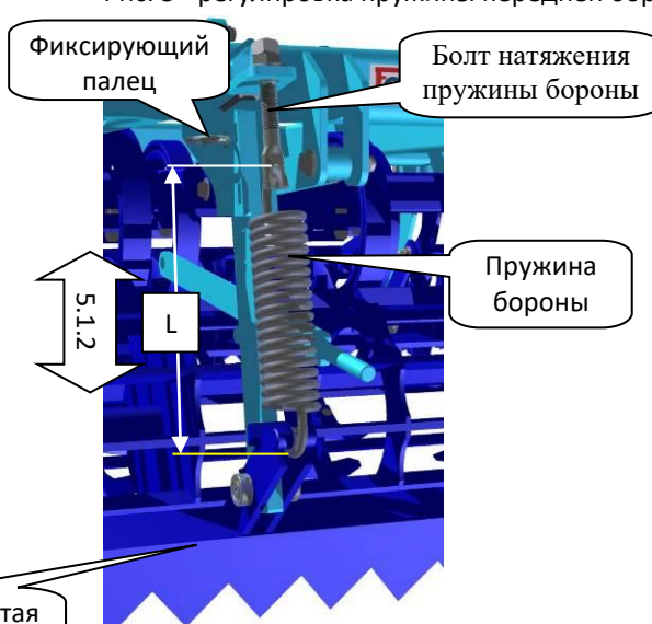
Рис. 5 - регулировка пружины передней бороны
