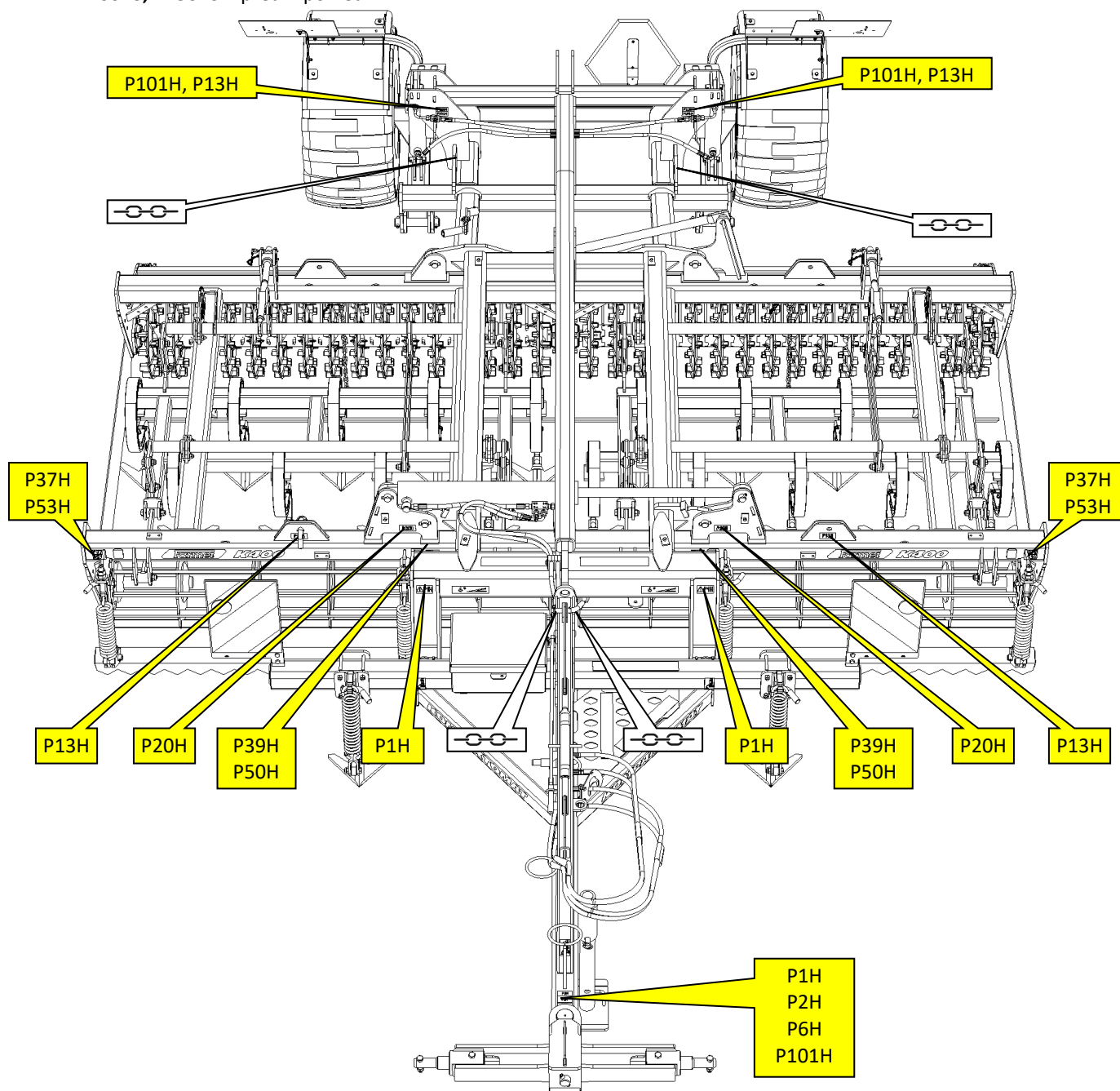
K400PS, K450PS – přední pohled
