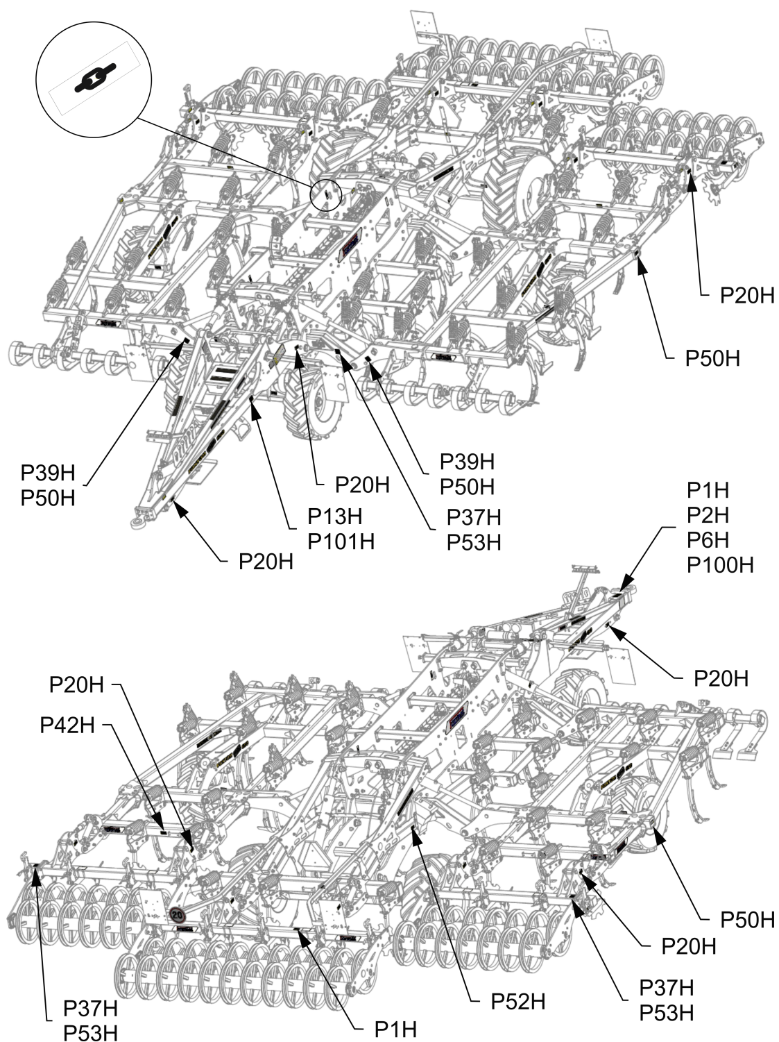
Рис.1 - Размещение предупредительных табличек на машине FANTOM 650 PRO, 800 PRO, 850 PRO FANTOM 650 PRO
