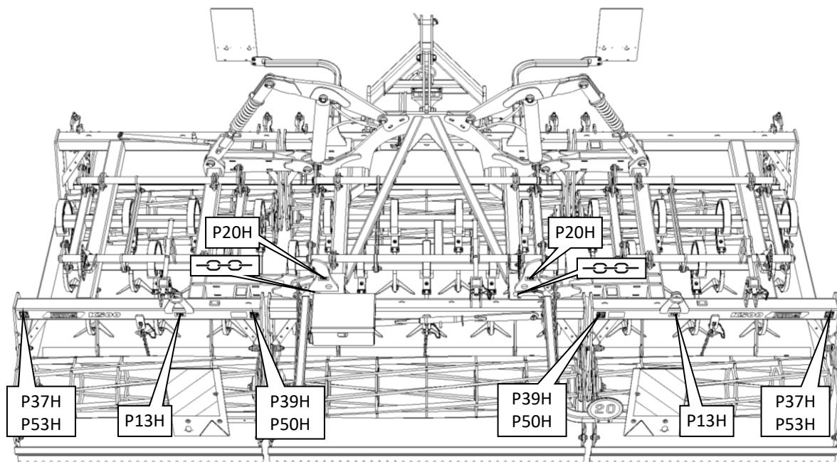
K500NS, K600NS - Rückansicht
