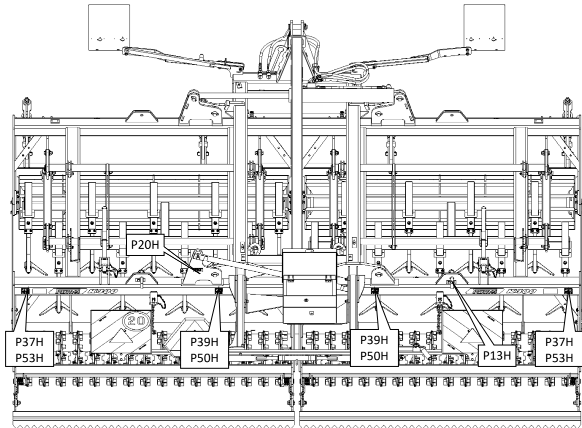
K400NS - Rückansicht
