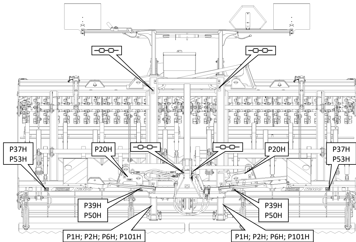
K400NS - Rückansicht
