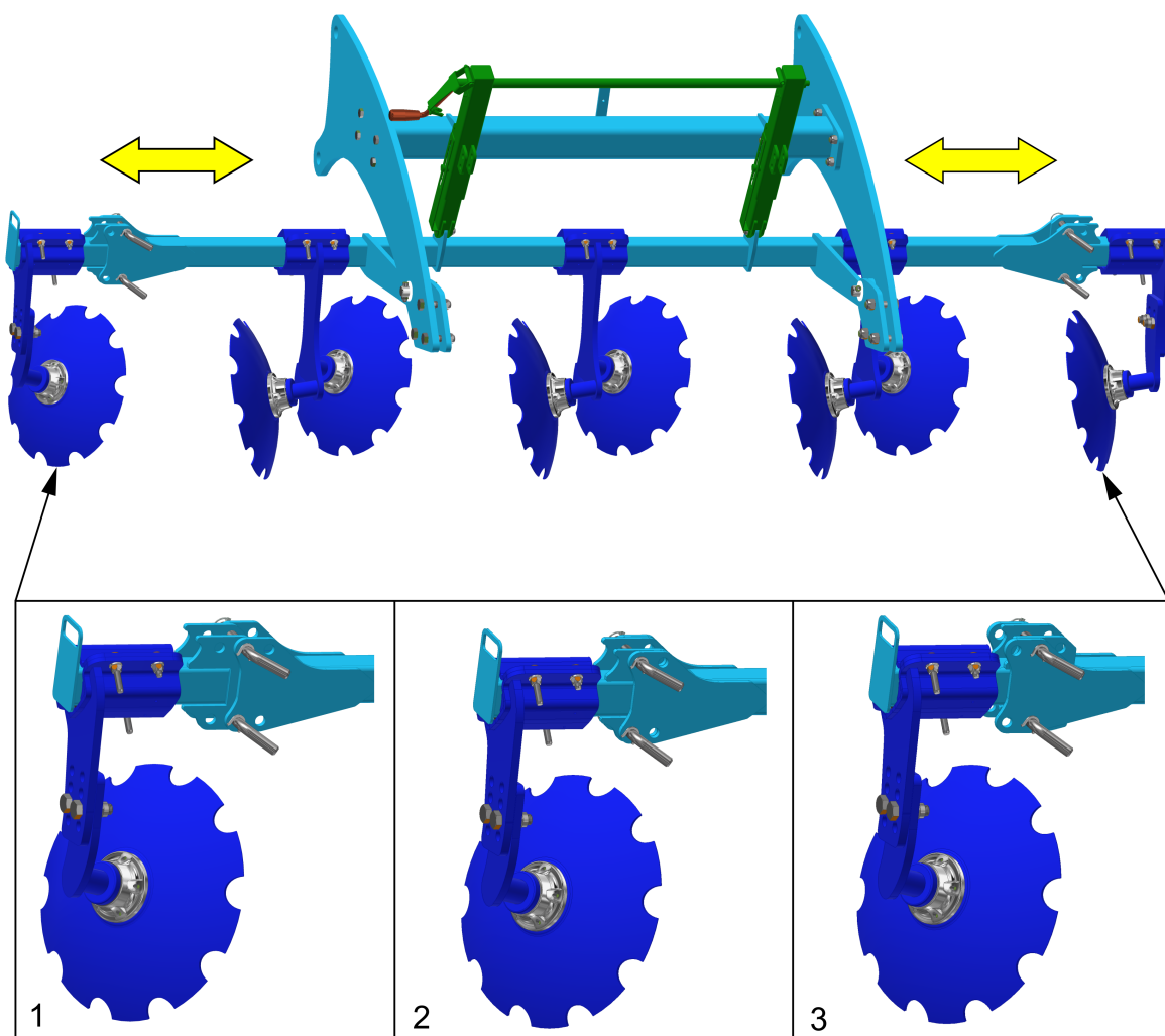
Rys. 9 - Regulowane wysokościowo dyski wyrównujące krawędzie
