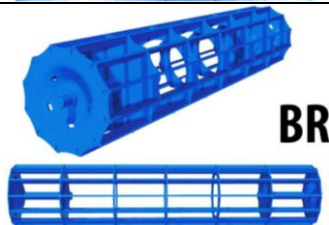
BR - rouleau à lames - Ø40 cm - 60 kg/m – 12 lattes
