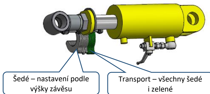
Obrázek 15 Podložky pístnice oje
