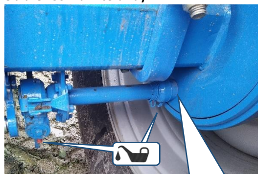
Obrázek 36 Maznice brzdy
