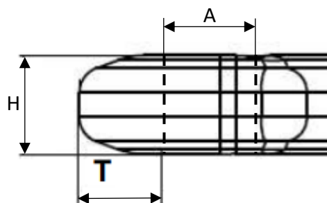
Obrázek 32 Kontrolované rozměry tažného oka
