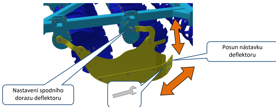
Obrázek 19 Možnosti nastavení bočních deflektorů
