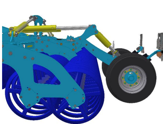
Obrázek 23 Poloha nápravy při otočce
