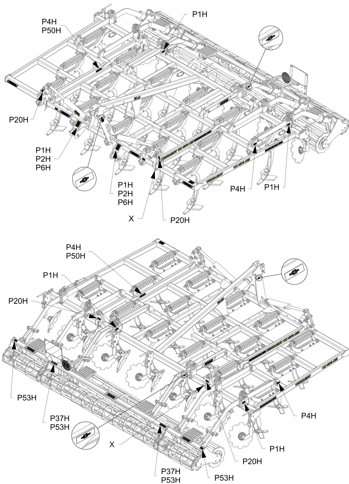
Рис.1 - Размещение предупредительных табличек на машине
