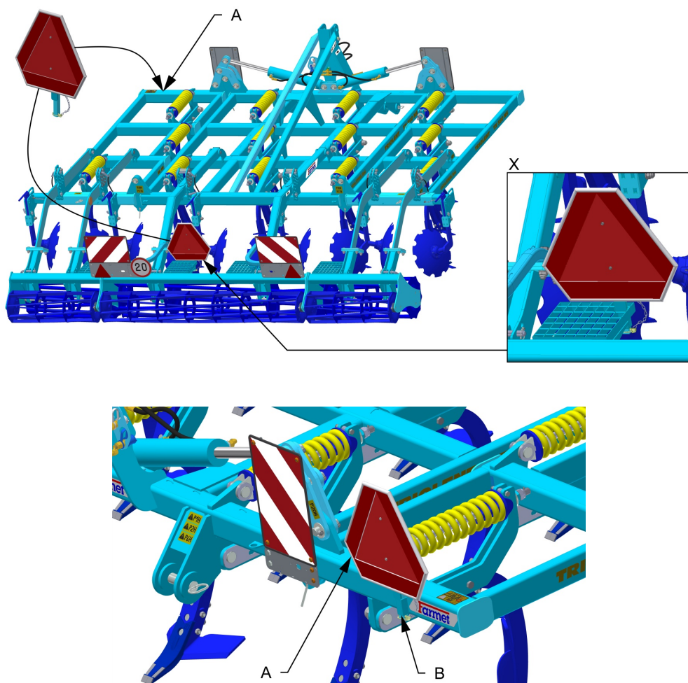
Рис.7 - размещение треугольника заднего обозначения транспортного средства с малой скоростью передвижения
