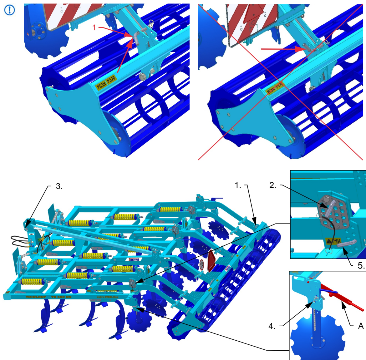
Рис.8 - порядок регулировки машины
