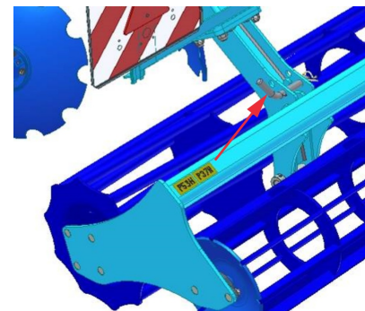
Рис.6 - задний двойной каток в трансп. положении
