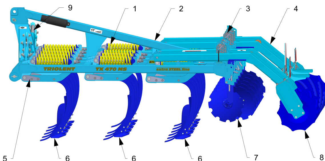
Рис.2 - РАБОЧИЕ УЗЛЫ МАШИНЫ
