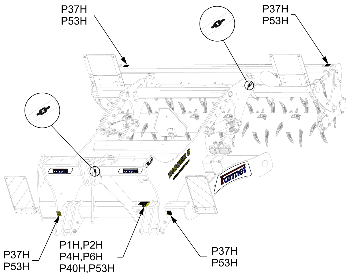
Рис.1 - Размещение предупредительных табличек на машине
