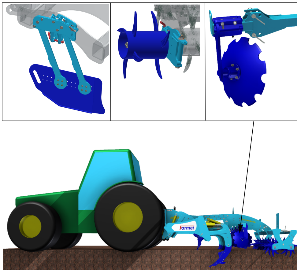
Рис.3 - Рабочее положение машины
