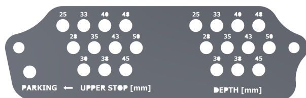
Деталь обозначения глубины
