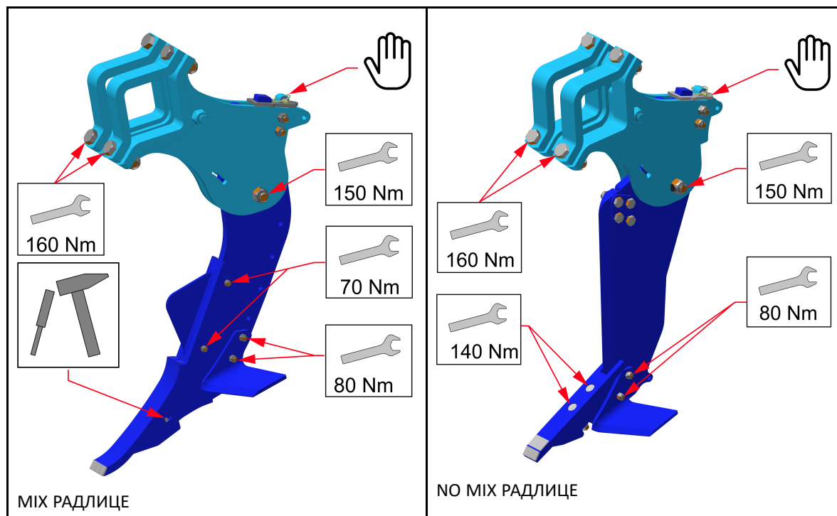
Рис.9 - замена быстроизнашивающихся деталей лапы
