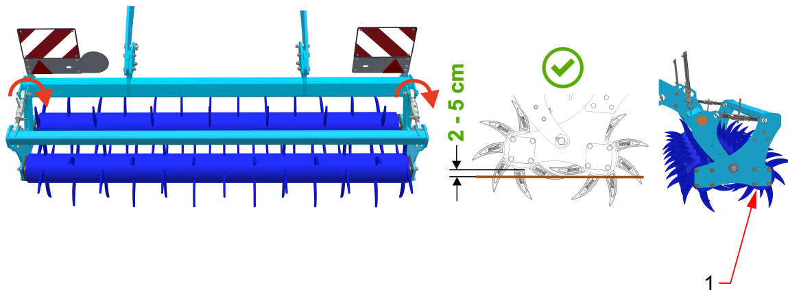
Рис.8 - изменение наклона катка
