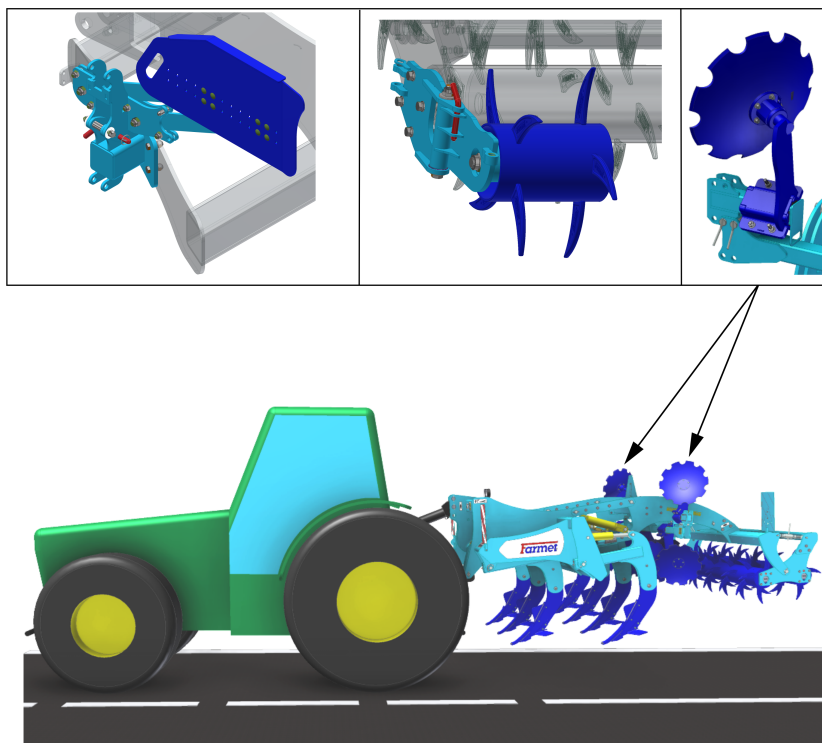
Рис.2 - транспортное положение машины
