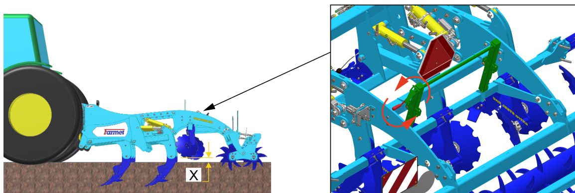
Рис.5 - установка положения дисков по высоте
