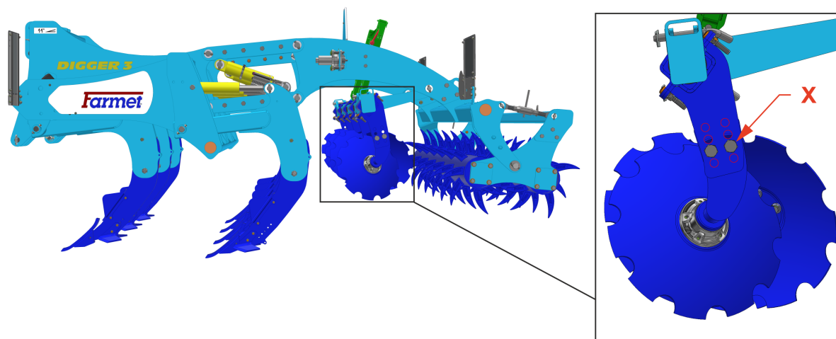
Рис.7 - Регулируемые по высоте краевые выравнивающие диски
