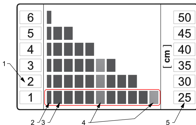
Рис.4 - комбинация подкладок для установки требуемой глубины
