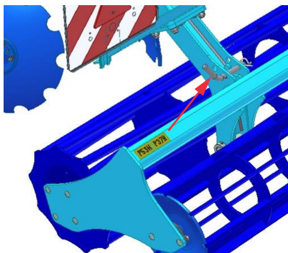
Rys. 6 - tylny podwójny walec w pozycji transportowej
