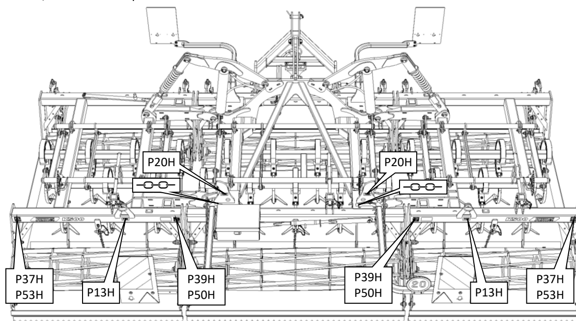
K500NS, K600NS - zadní pohled
