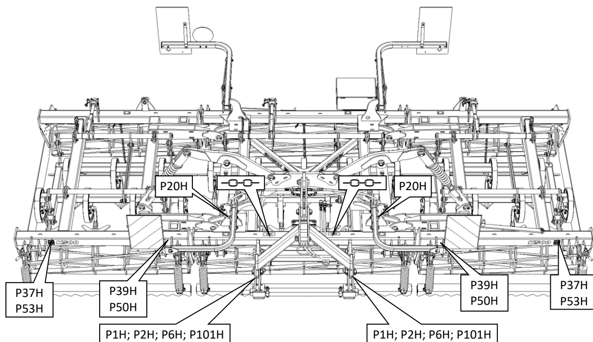
K500NS, K600NS - přední pohled
