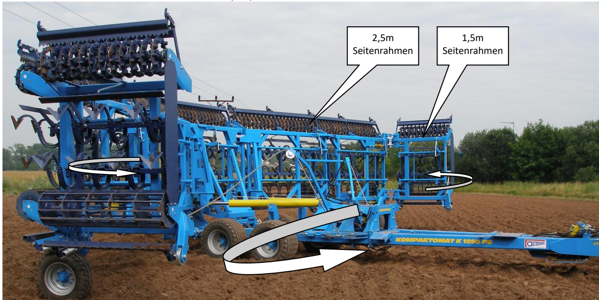
Abb. 15 - Schließen der Arbeitssektionen in die Transportposition
