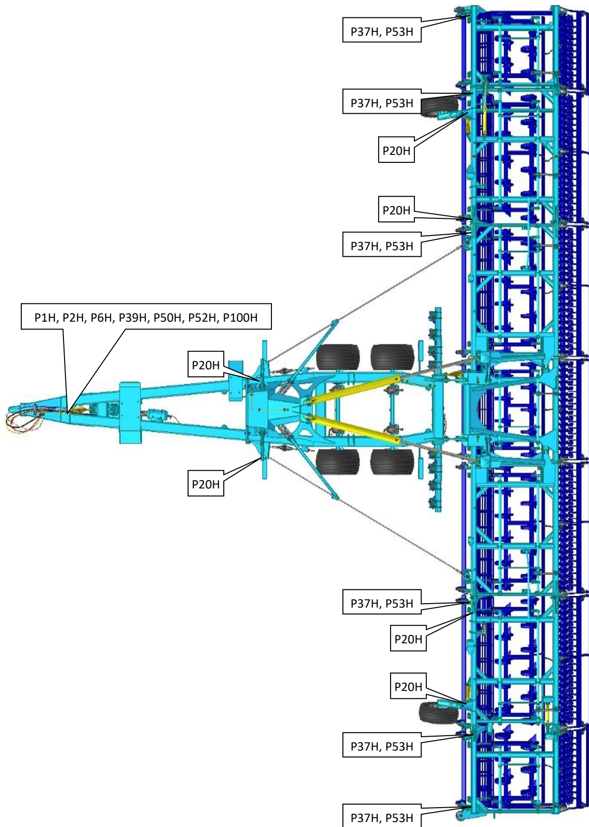
Abb. 1: Befestigungsstellen der Warnbildzeichen und Hinweisschilder an dem K 1250 PS, K 1570 PS
