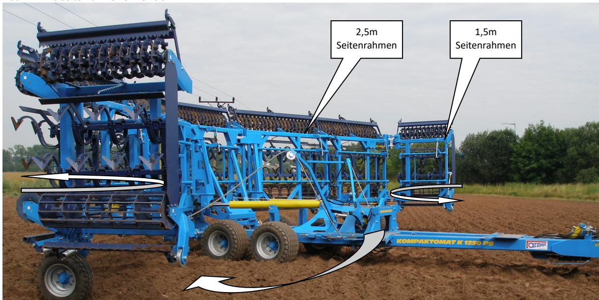
Abb. 11 - Die Seitenrahmen öffnen sich
