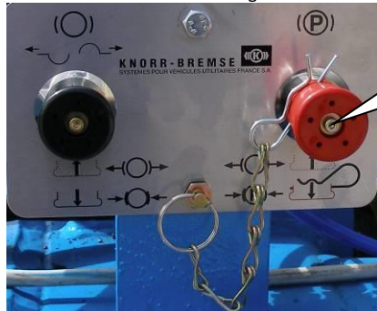
Abb.28-Detail der Beschreibung der Ventilbedienung der Bremsen
