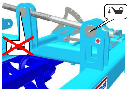
Abb.32 - Kurbel
