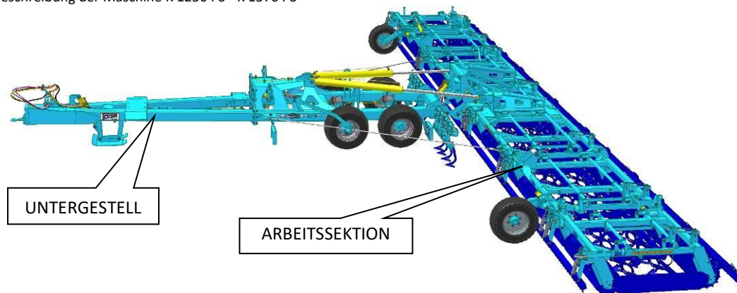
Abb. 2: Beschreibung der Maschine K 1250 PS - K 1570 PS
