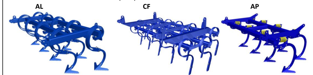
VARIANTEN DER SCHARSEKTIONEN (S.14)
