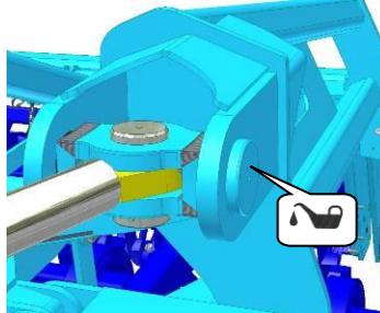
Abb. 33 - Lager der Kolbenstangenlagerung
