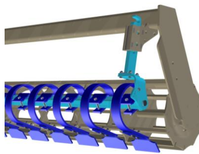
L+FB-С ЛОПАТКАМИ
